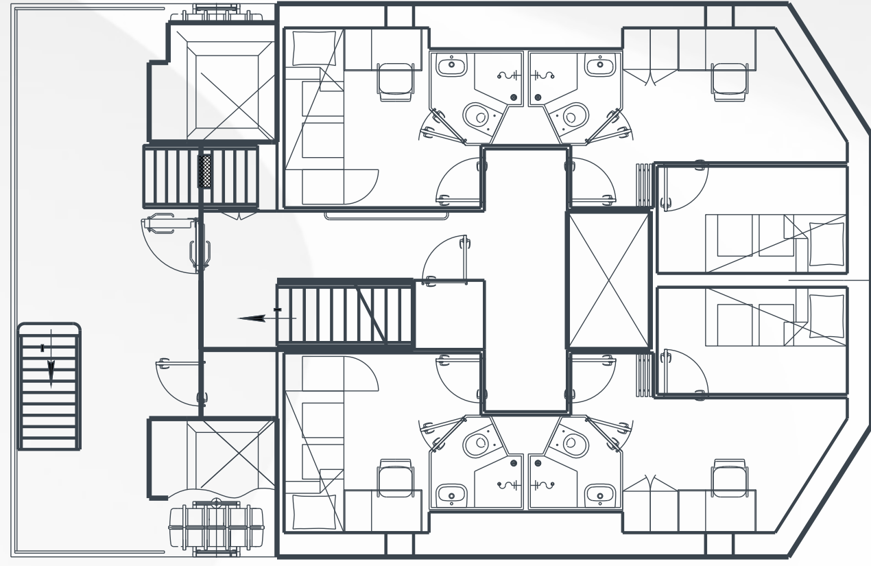
Палуба надстройки (1 ярус)
